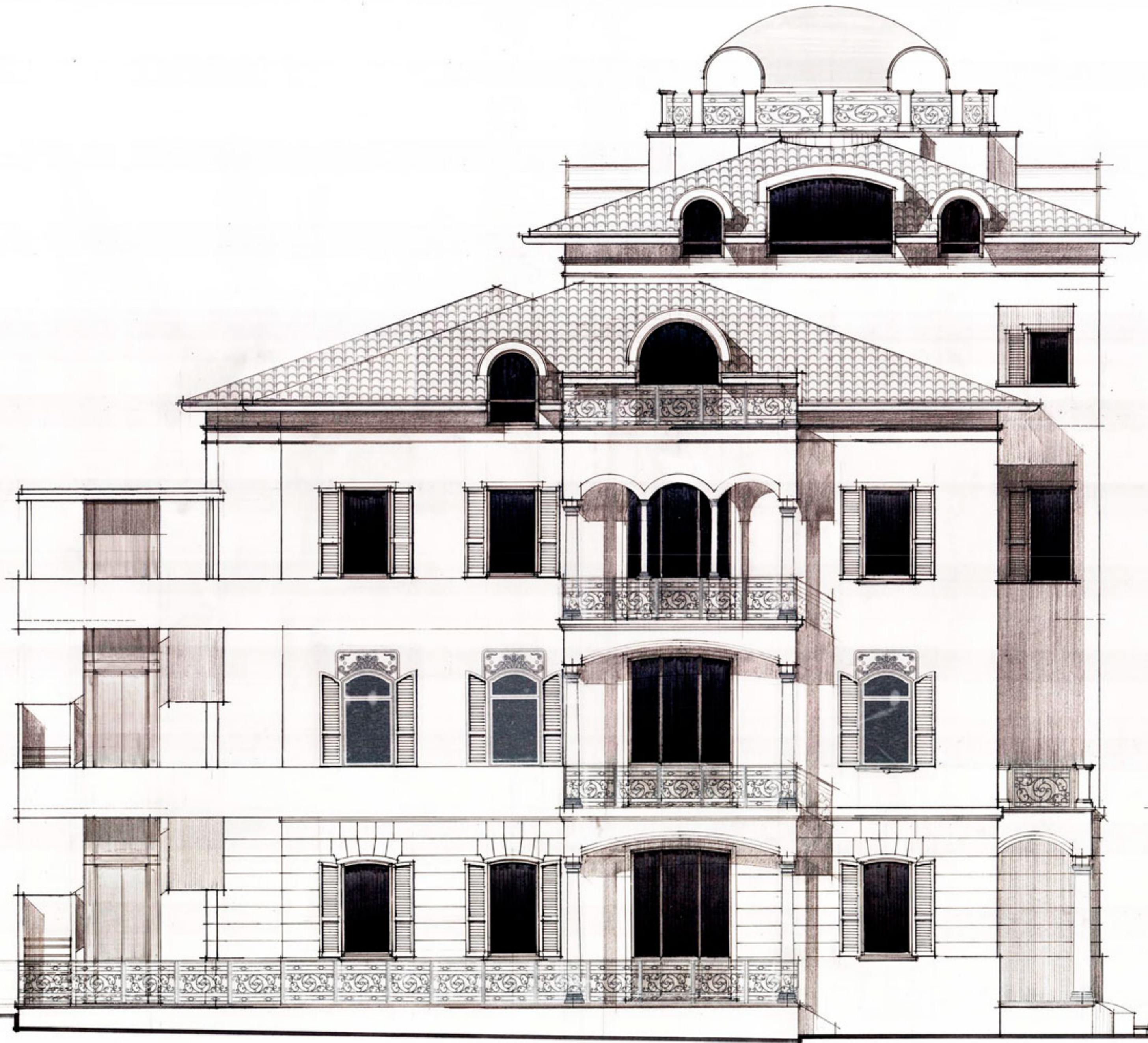
VILLA CASATI CONFALONIERI - PROSPETTO NORD/OVEST
